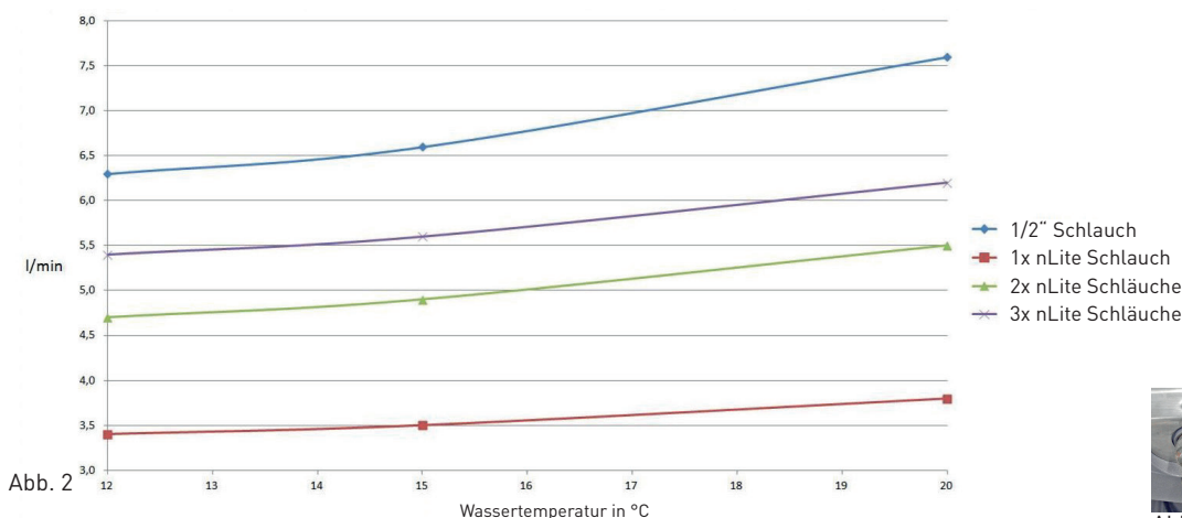
Abb. 2 Abhängigkeit der Leistung von Wassertemperatur und Schlauchdurchmesser bzw. Anzahl der Schläuche. Abb. 2a Der rechte Wasseranschluß erhält mehr Wasser von den Membranen als der Mittlere oder der Linke. Daher sollten längere Schläuche oder höhere Stangen rechts angeschlossen werden.
