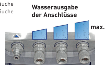
Abb. 2 Abhängigkeit der Leistung von Wassertemperatur und Schlauchdurchmesser bzw. Anzahl der Schläuche. Abb. 2a Der rechte Wasseranschluß erhält mehr Wasser von den Membranen als der Mittlere oder der Linke. Daher sollten längere Schläuche oder höhere Stangen rechts angeschlossen werden.
